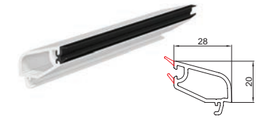
20 MM ÇİFT CAM ÇITA PROFİLİ
